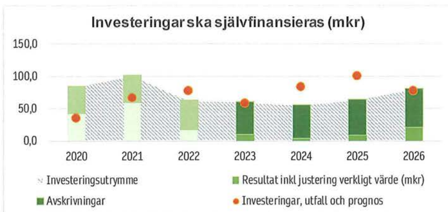
Diagram 2: visar investeringsutrymmet jämfört med investeringsplanen över tid.
